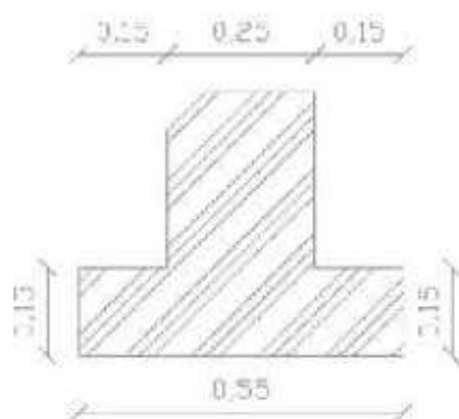
Εικόνα: Διατομή κρασπέδου που τοποθετείται στην περίμετρο της στρώσης διαβαθμισμένης άμμου
