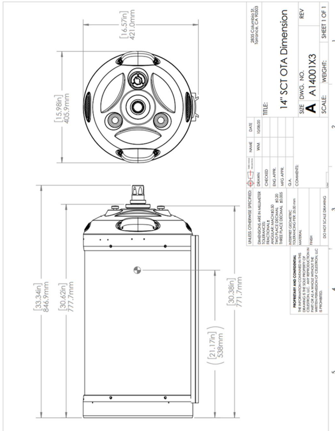
Σχέδιο Οπτικού Σωλήνα διαμέτρου 14"
