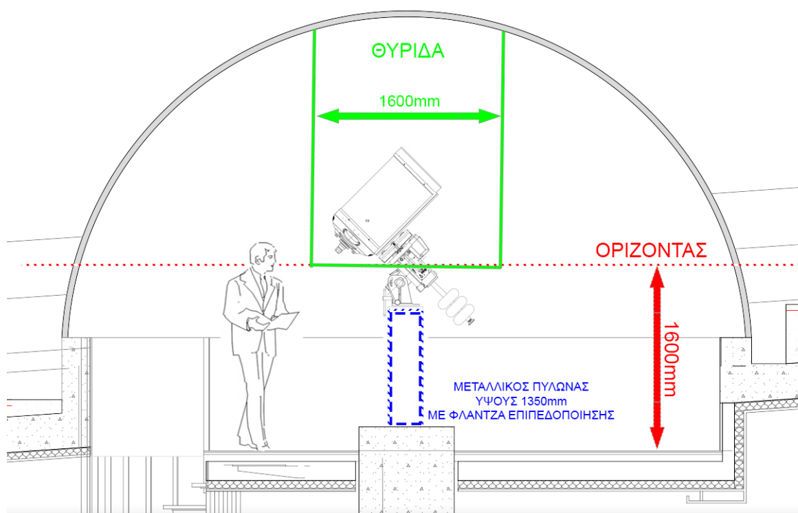
Ενδεικτικό Σχέδιο Θόλου Αστεροπαράτηρησης
